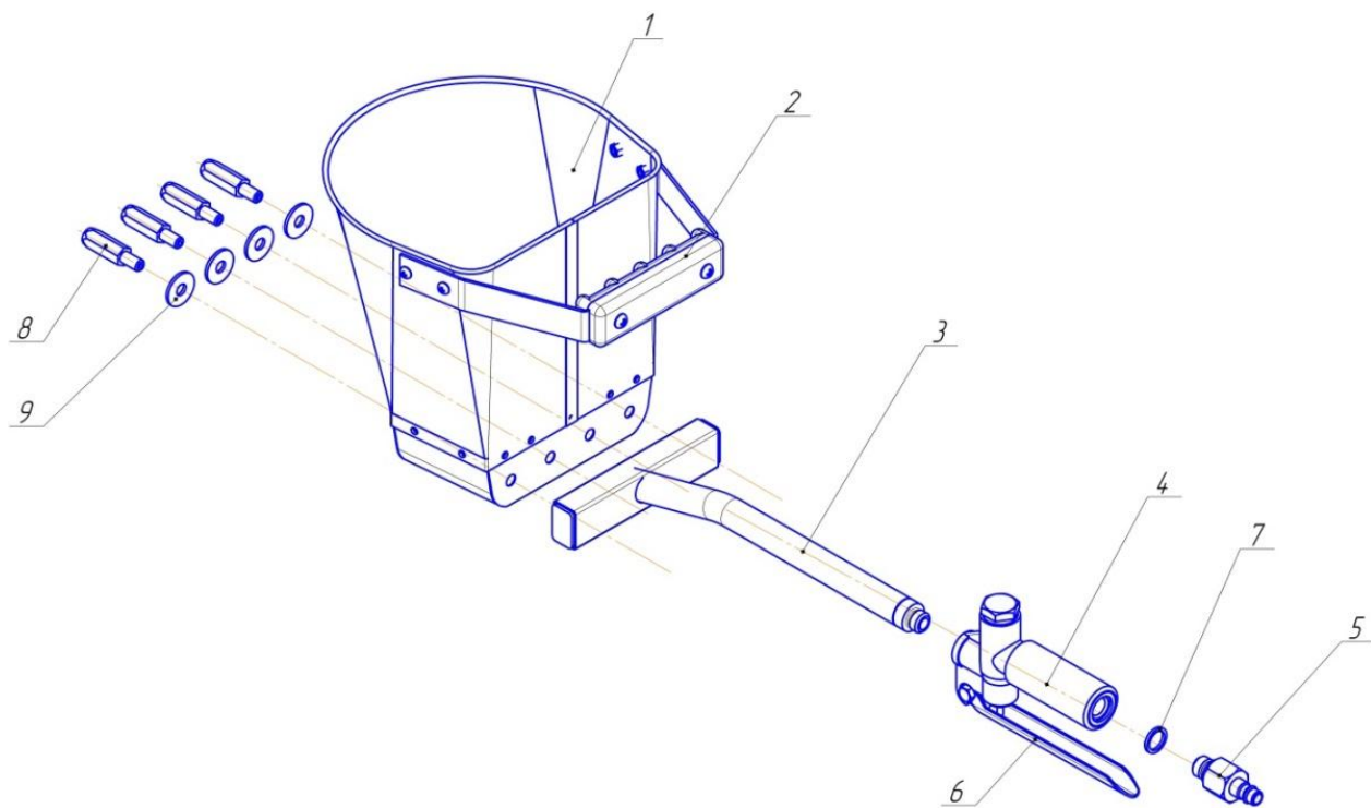
Рис.1 Основные составные части ковша штукатурного:
